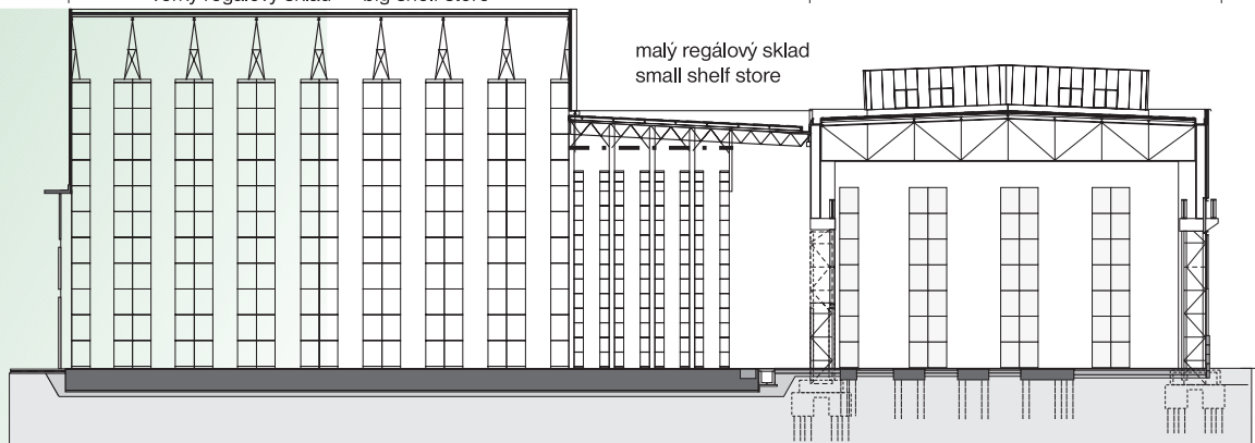
OBJEKT 005 OBJEKT 001 PRIEČNY REZ A - A' CROSS - SECTION A - A' OBJEKT 004
